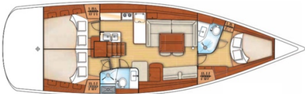
BENETEAU OCEANIS 46 ( 3 Cabins)
